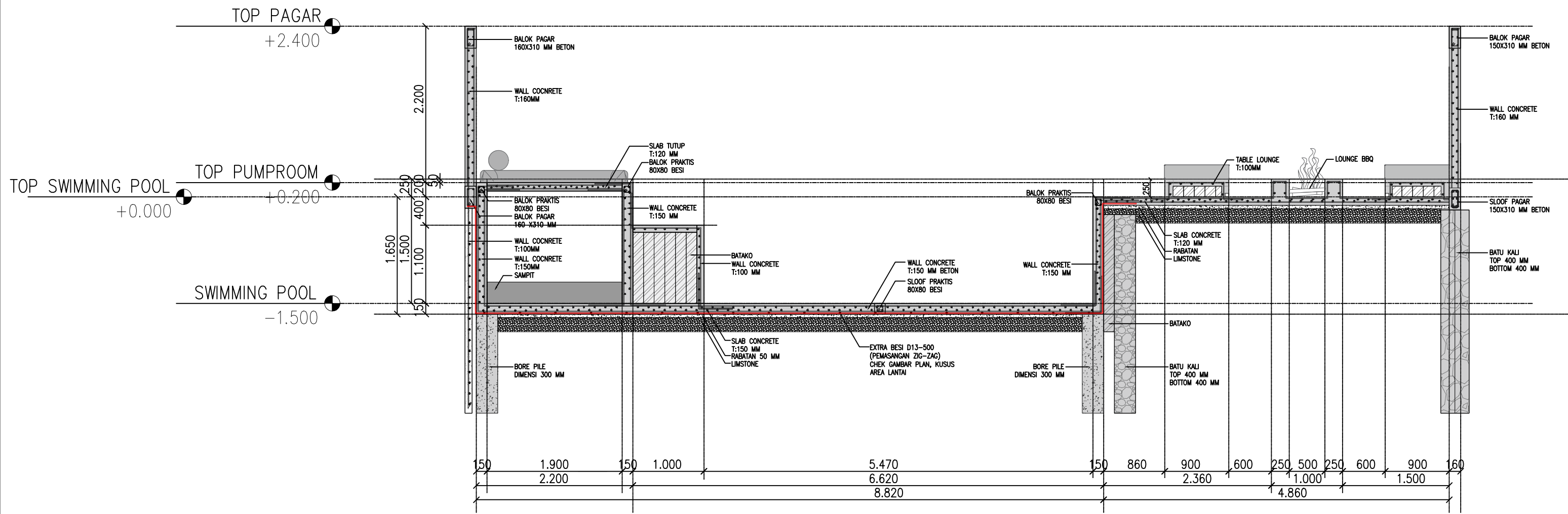
○ KABAKABA CASCADE. SECTION B 1 : 100
