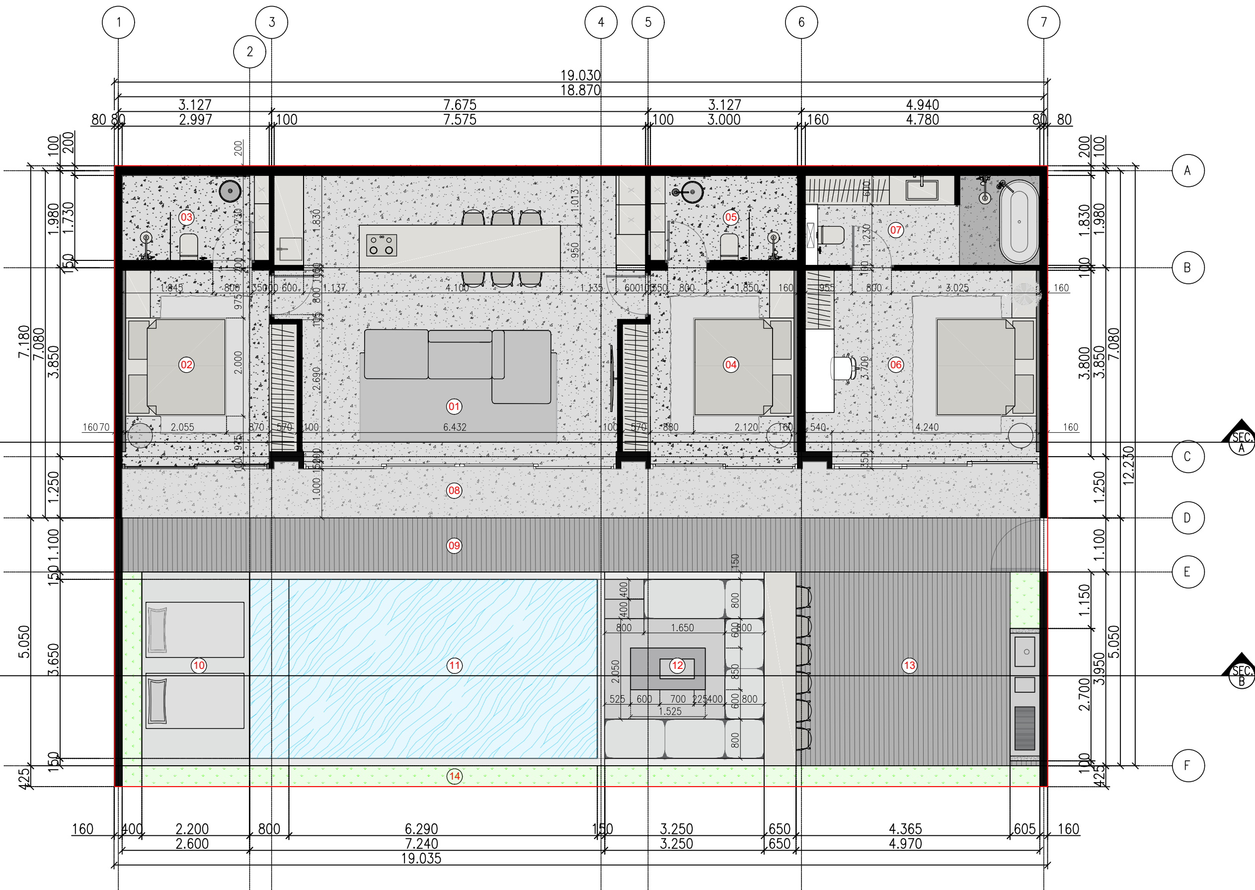
KABAKABA CASCADE. VILLA 3BR PLAN 1:100
