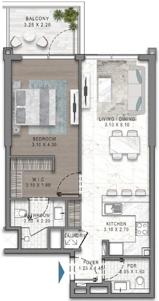
1BR - TYPE K3
