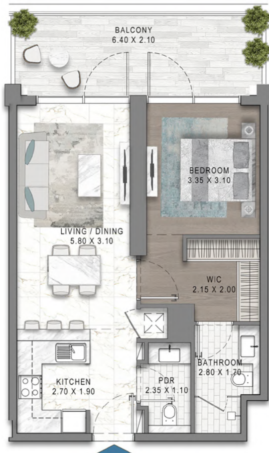
1BR - TYPE A11
