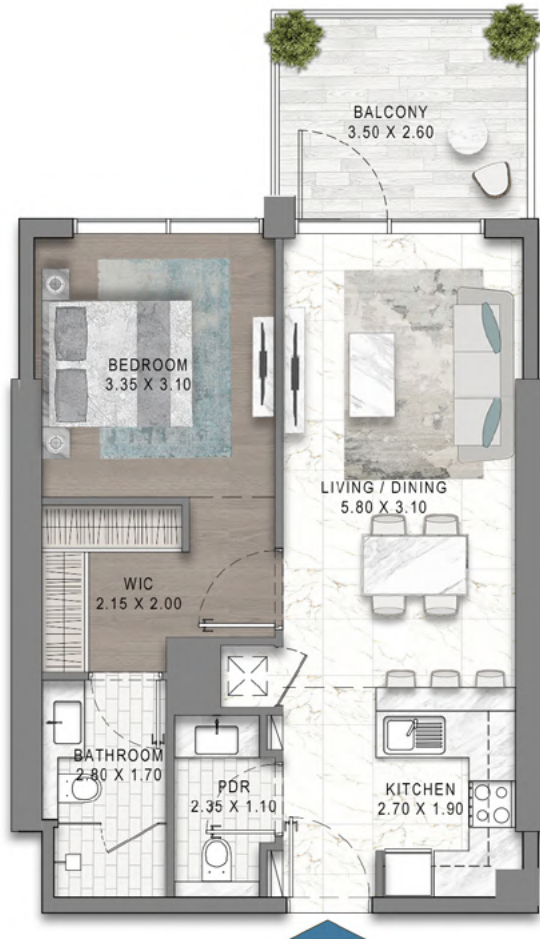
1BR - TYPE A15
