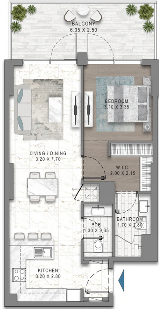
1BR - TYPE E1
