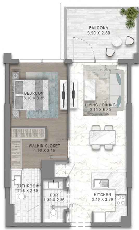
1BR - TYPE F4
