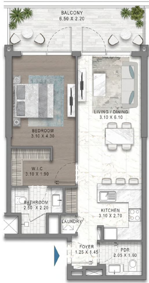
1BR - TYPE K1
