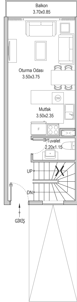
ZEMİN KAT
