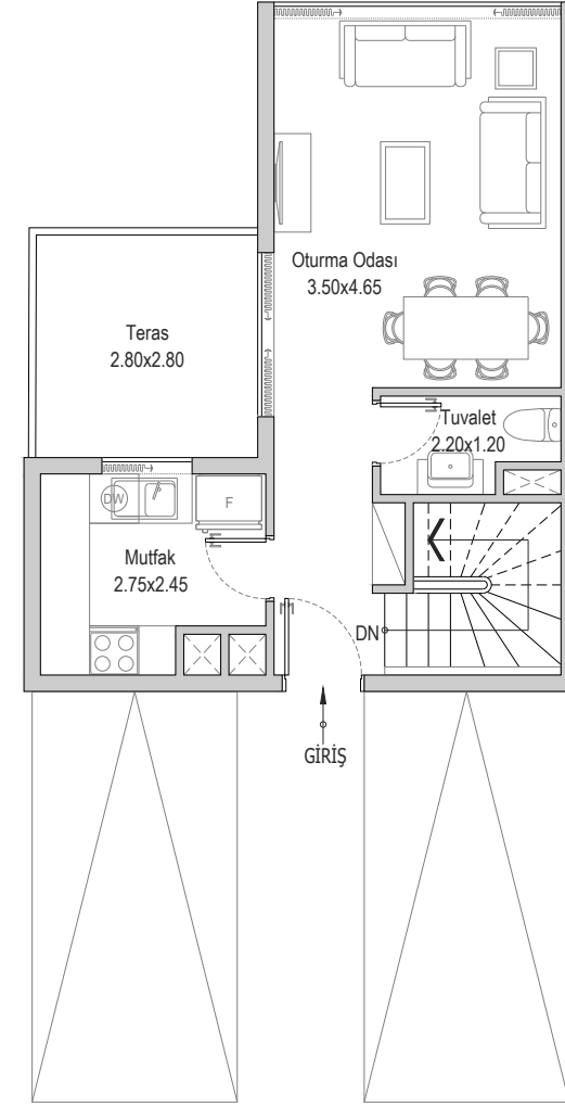
ZEMİN KAT
