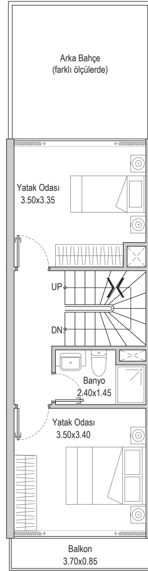
BİRİNCİ KAT
