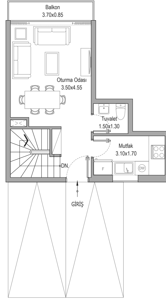
ZEMİN KAT
