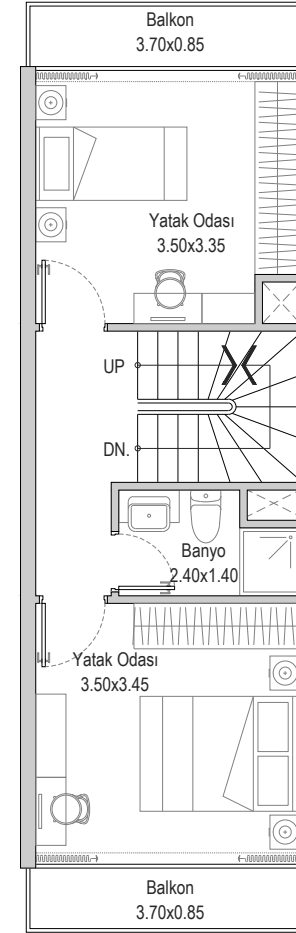
İKİNCİ KAT
